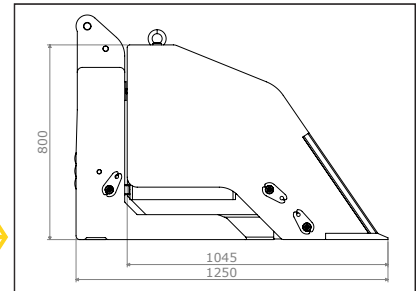
↑ HydroTwin frameaanzicht.
