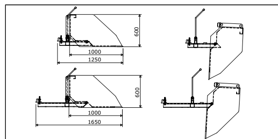
↑ Heftruckbakken mechanisch doorsteek en dicht
