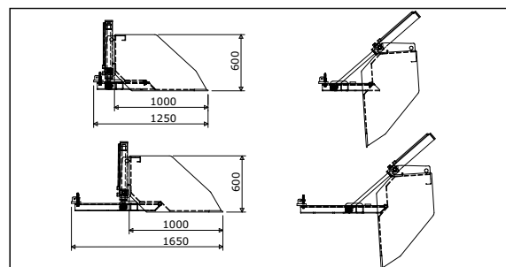
↑ Heftruckbakken hydraulisch doorsteek en dicht
