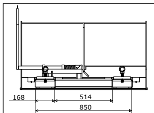
↑ Afmetingen Lepelkokers voor alle uitvoeringen.
