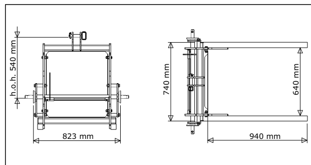
↑ Palletdrager C-2
