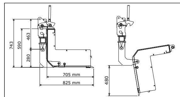
↑ Mechanische Trekkerbak C-0
