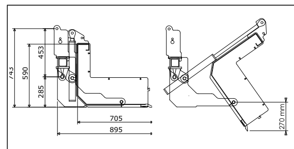
↑ Hydraulische Trekkerbak C-0
