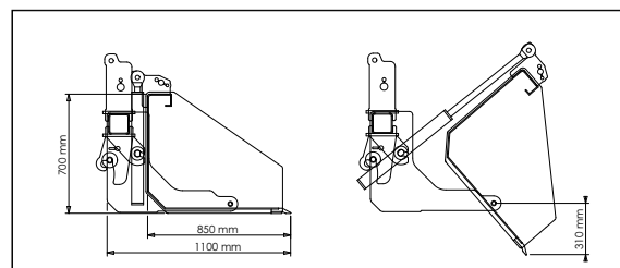
↑ Hydraulische Trekkerbak C2
