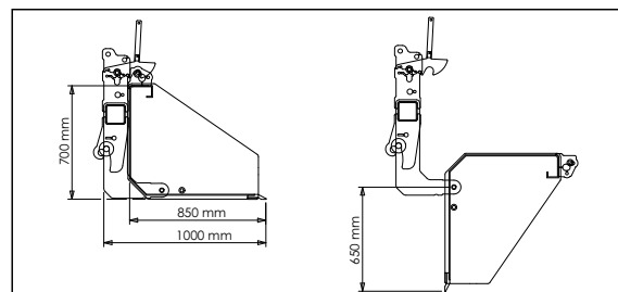
↑ Mechanische Trekkerbak C2
