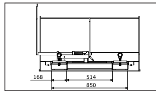
↑ Afmetingen Lepelkokers voor alle uitvoeringen.
