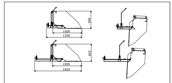
↑ Heftruckbakken mechanisch doorsteek en dicht
