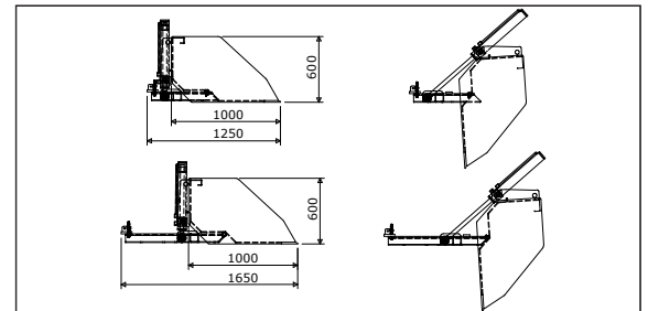
↑ Heftruckbakken hydraulisch doorsteek en dicht
