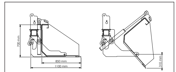
↑ Hydraulische Trekkerbak C2
