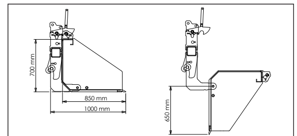
↑ Mechanische Trekkerbak C2
